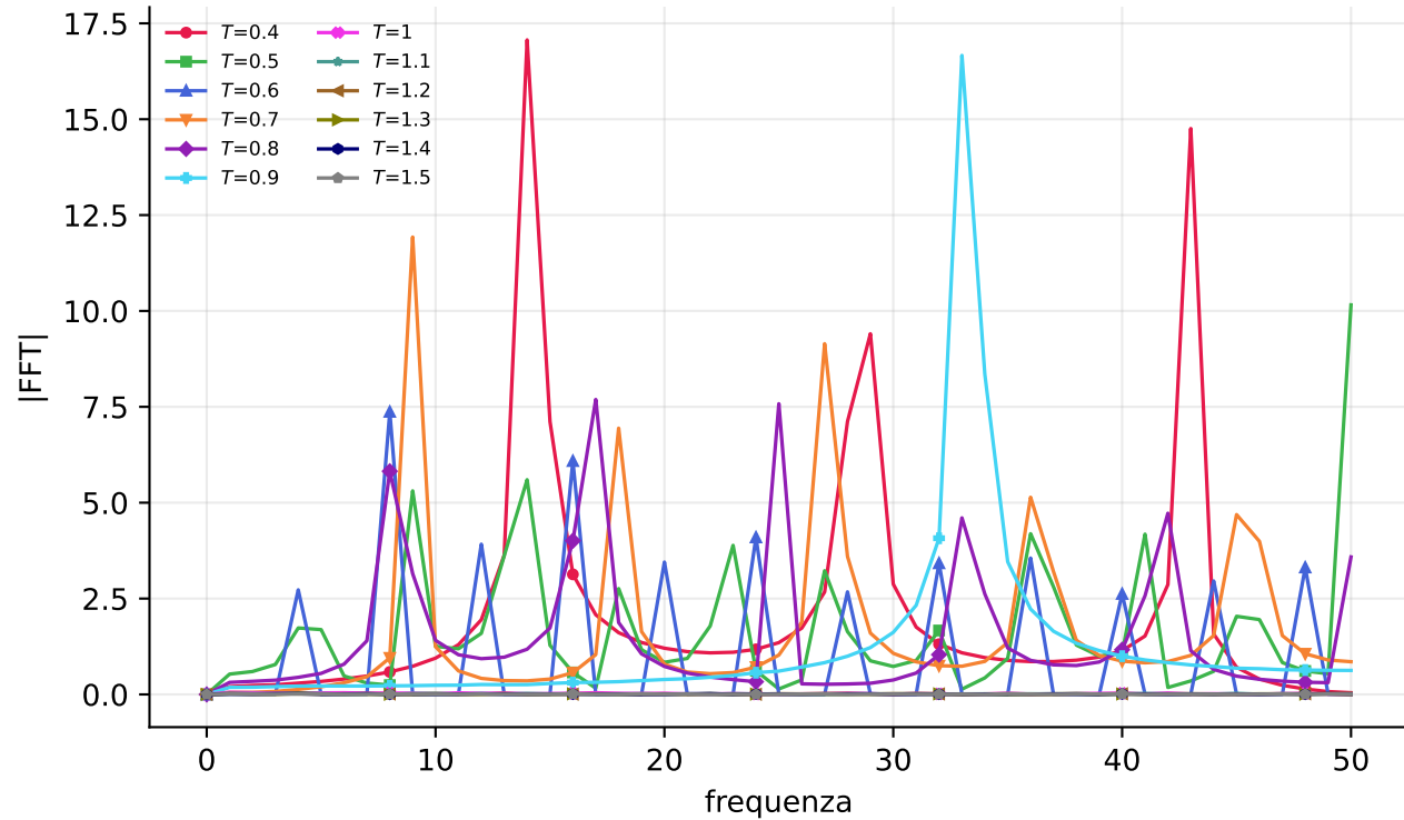
Trasformata dell'ACF: i picchi sono la fase periodica
